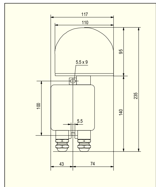
Obelux 10-115-F dimensions
